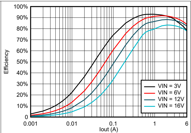
图 6-14. TPS566247 在 1.05V_{OUT} 且使用 1\mu H 电感器时的效率
