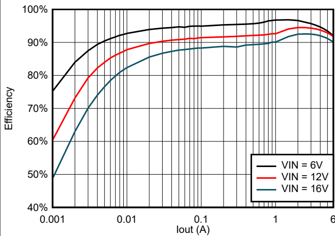
图 6-15. TPS566242 在 3.3V_{OUT} 且使用 2.2\mu H 电感器时的效率
