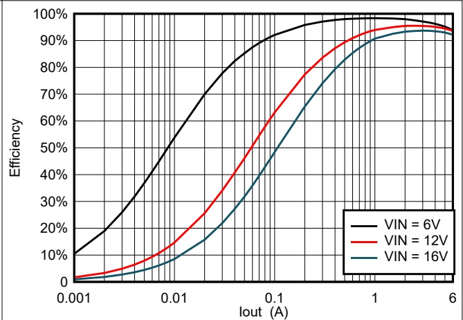
图 6-18. TPS566247 在 5V_{OUT} 且使用 2.2\mu H 电感器时的效率
