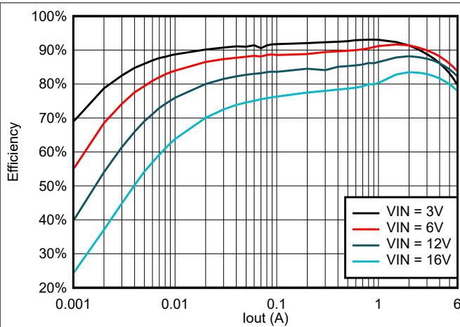
图 6-13. TPS566242 在 1.05V_{OUT} 且使用 1\mu H 电感器时的效率
