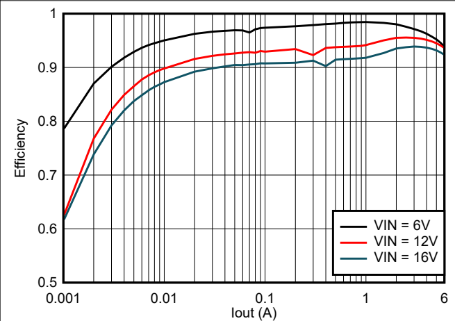
图 6-17. TPS566242 在 5V_{OUT} 且使用 2.2\mu H 电感器时的效率
