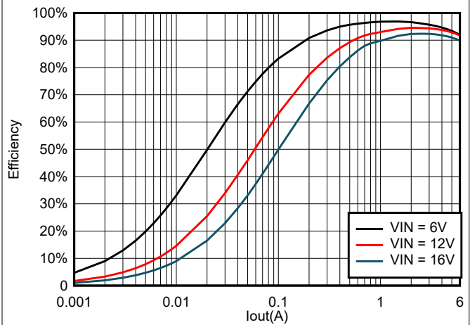
图 6-16. TPS566247 在 3.3V_{OUT} 且使用 2.2\mu H 电感器时的效率
