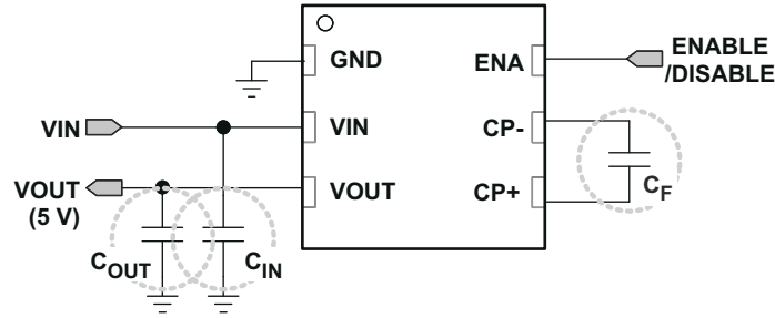
图 7-2. 电容器
