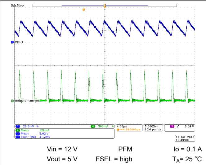
图 10-57. Output Voltage Ripple
