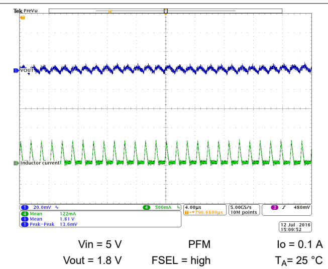
图 10-43. Output Voltage Ripple
