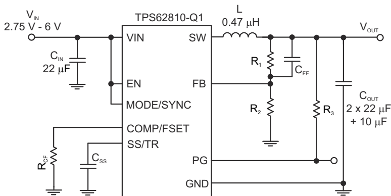
图 9-1. 典型应用
