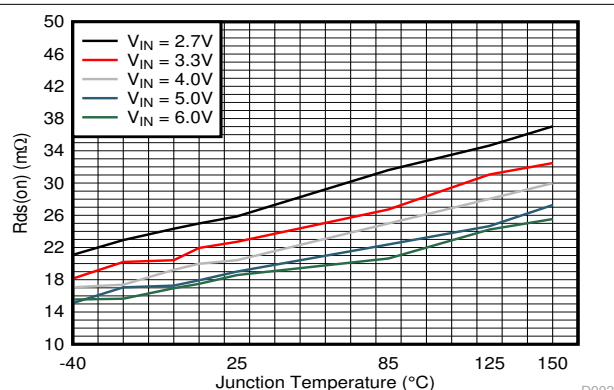
图 6-2. 低侧开关的 R_{ds(on)}
