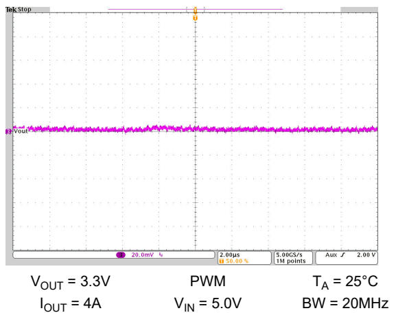
图 9-43. 输出电压纹波
