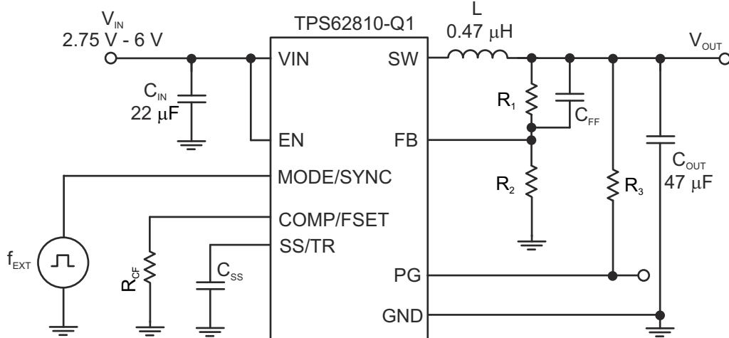
图 9-60. 使用外部同步的原理图
