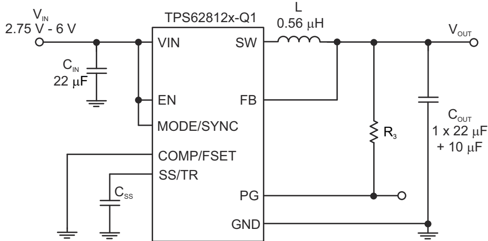
图 9-57. 固定输出电压版本的原理图
