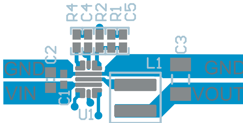
图 9-63. 示例布局
