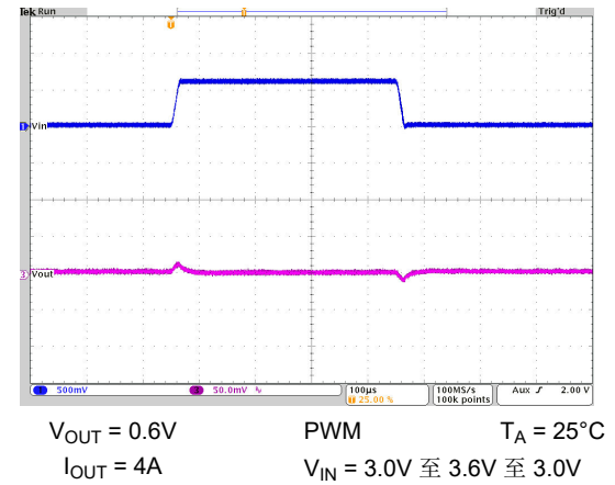
图 9-41. 线路瞬态响应
