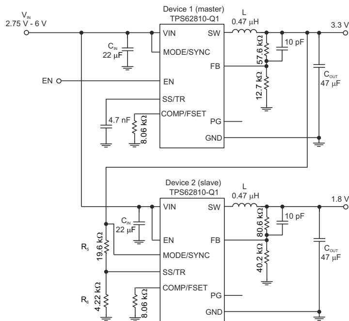
图 9-58. 输出电压跟踪原理图
