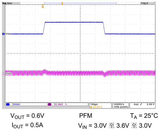
图 9-40. 线路瞬态响应
