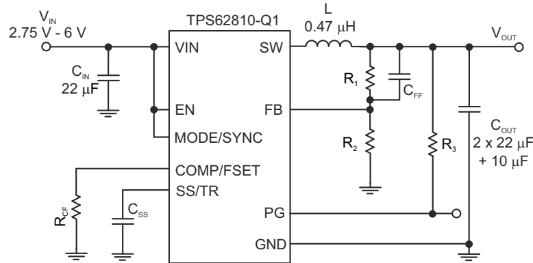
图 7-1. TPS62810-Q1 和 TPS62813-Q1 的测量设置
