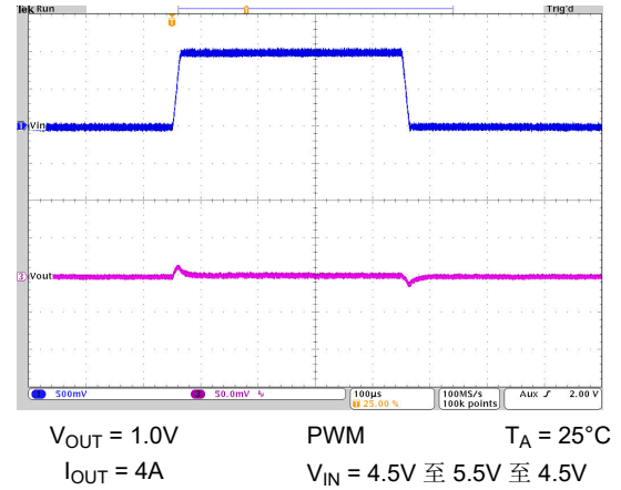
图 9-39. 线路瞬态响应
