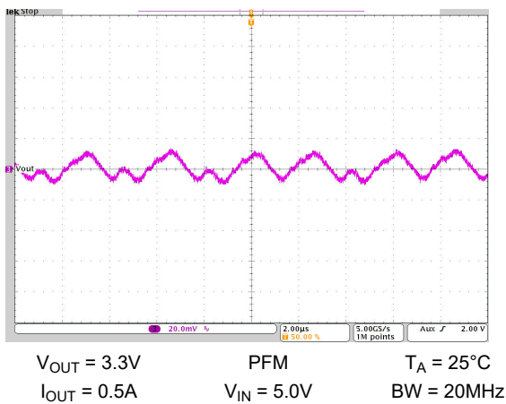
图 9-42. 输出电压纹波
