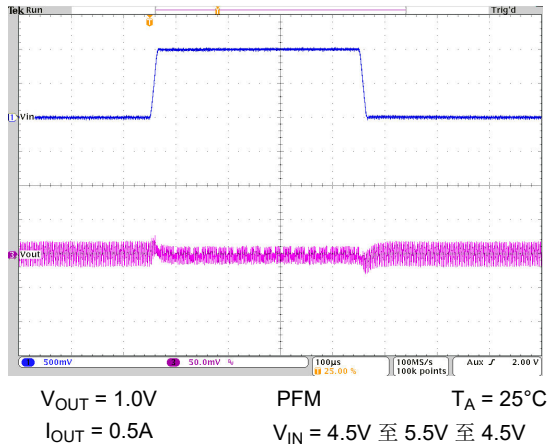
图 9-38. 线路瞬态响应
