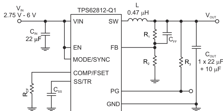
图 7-2. TPS62812-Q1 和 TPS62811-Q1 的测量设置
