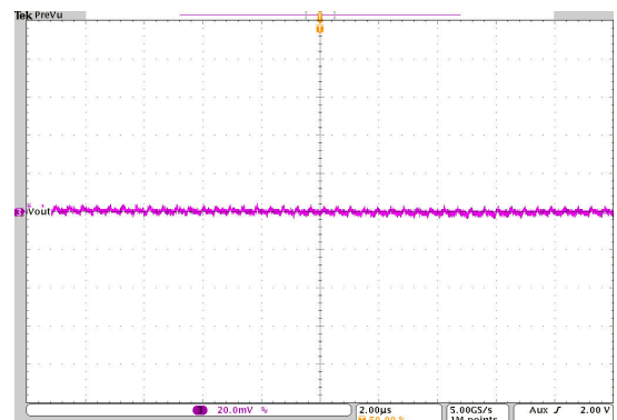
图 10-47. Output Voltage Ripple
