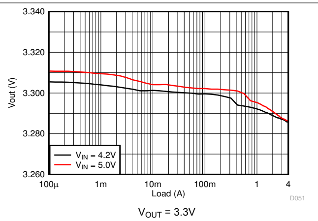
图 8-20. Load Regulation
