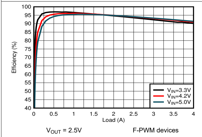
图 8-17. PWM Efficiency
