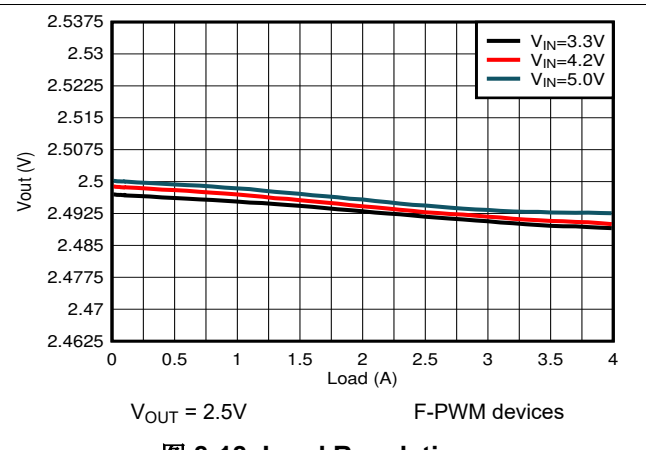
图 8-18. Load Regulation
