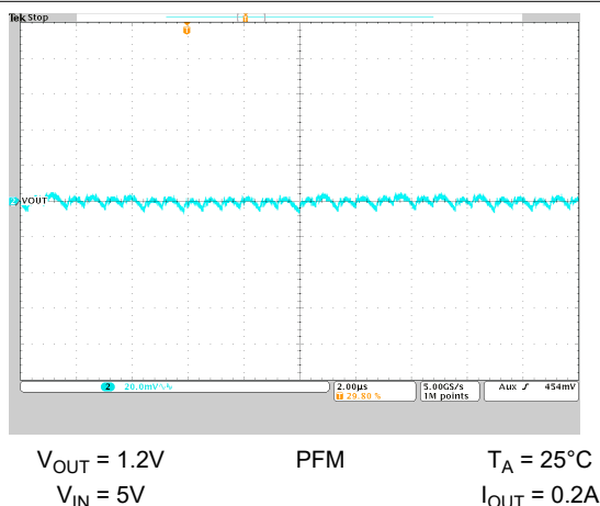
图 9-46. 输出电压纹波
