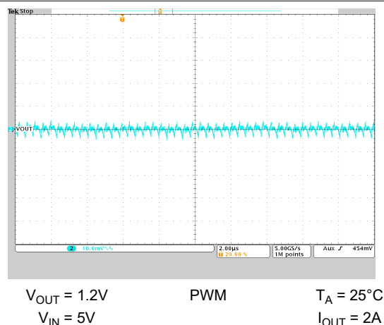
图 9-47. 输出电压纹波
