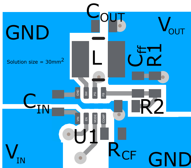
图 9-60. 示例布局
