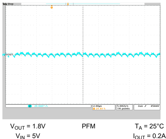
图 9-44. 输出电压纹波
