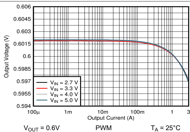
图 9-17. 输出电压与输出电流间的关系
