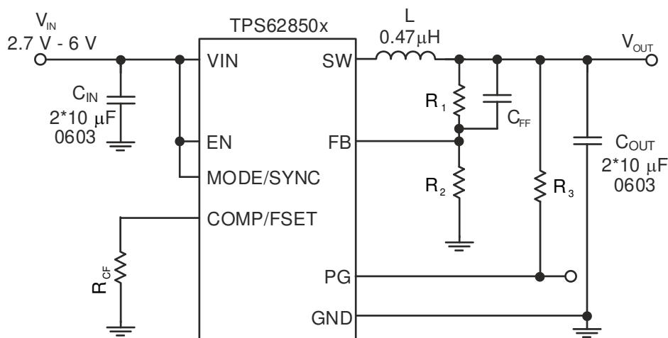
图 9-1. 典型应用
