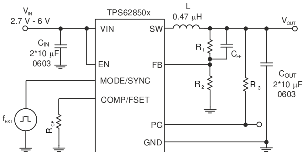
图 9-57. 使用外部同步的原理图
