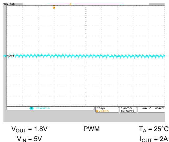
图 9-45. 输出电压纹波
