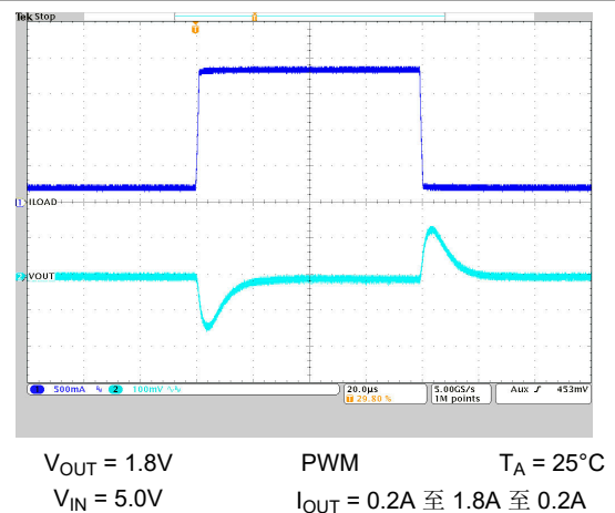
图 9-25. 负载瞬态响应
