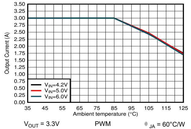
图 9-21. 输出电流与环境温度间的关系
