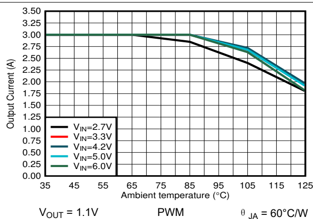
图 9-19. 输出电流与环境温度间的关系
