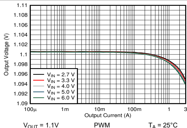
图 9-15. 输出电压与输出电流间的关系
