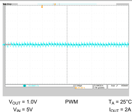
图 9-49. 输出电压纹波
