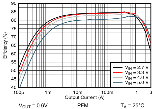
图 9-8. 效率与输出电流间的关系
