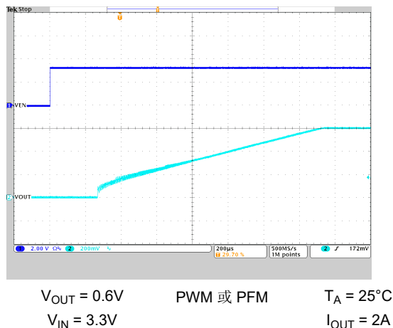
图 9-56. 启动时序
