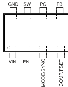
图 5-1. 8 引脚 SOT583 DRL 封装 (顶视图)
