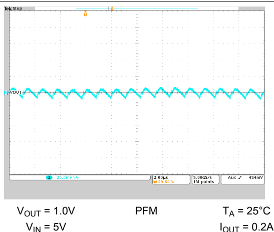
图 9-48. 输出电压纹波
