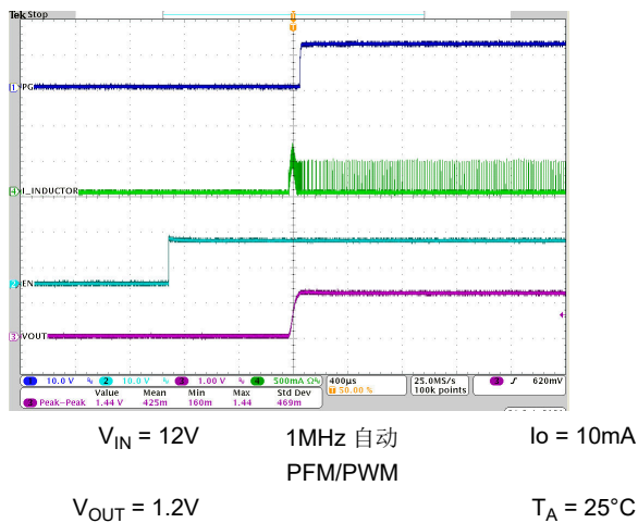
图 7-41. 启动时序
