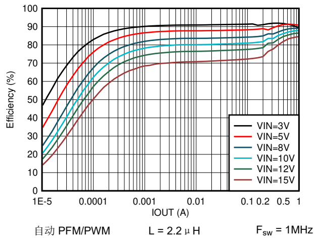
图 7-19. 效率与输出电流间的关系 V OUT = 1.2V
