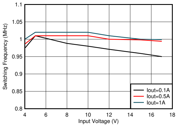
图 7-26. 开关频率与输入电压间的关系 V_{OUT} = 5V
