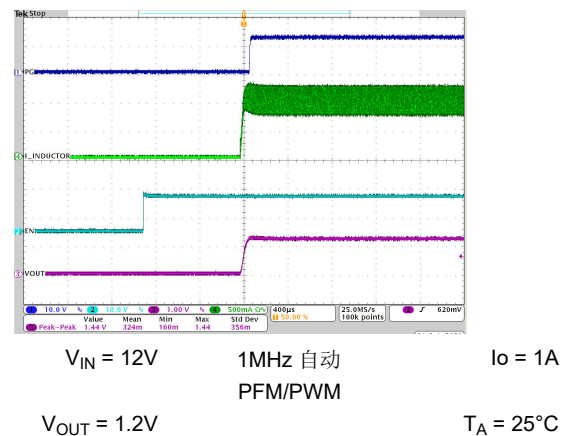
图 7-42. 启动时序
