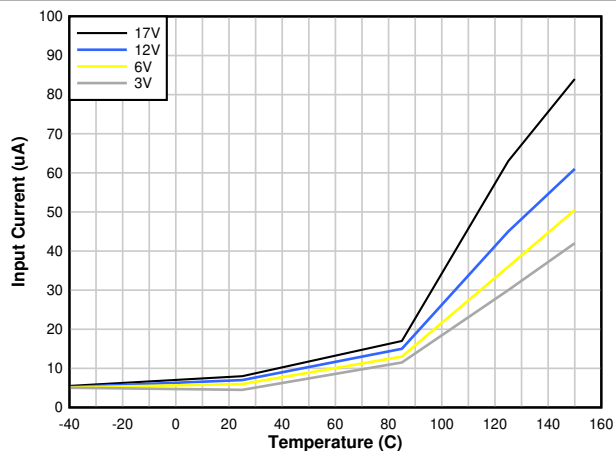
图 5-2. 最大静态电流与温度间的关系
