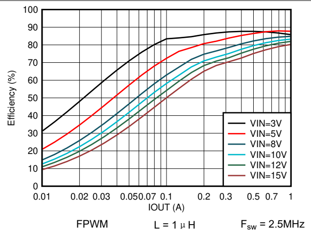
图 7-22. 效率与输出电流间的关系 V OUT = 1.2V
