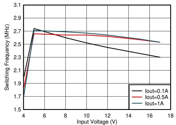
图 7-28. 开关频率与输入电压间的关系 V_{OUT} = 3.3V
