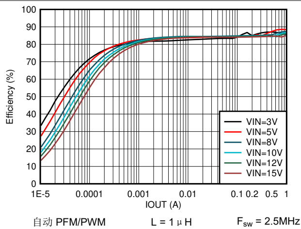
图 7-21. 效率与输出电流间的关系 V OUT = 1.2V
