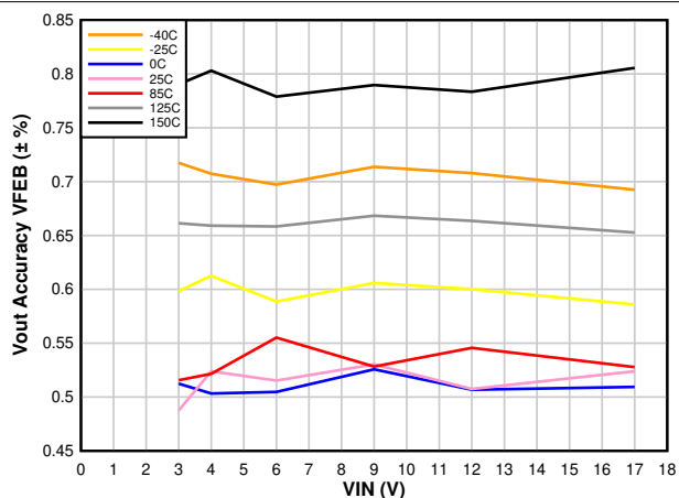
图 5-4. 输出电压精度 - 选择 VFEB
