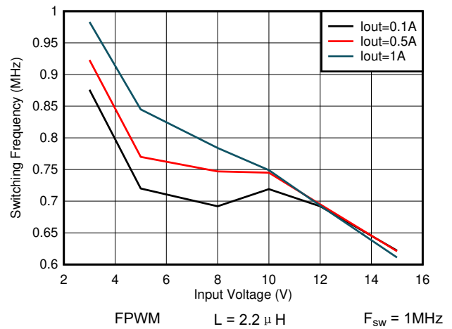
图 7-74. 开关频率与输入电压间的关系 V_{OUT} = 0.4V
