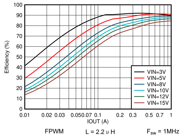
图 7-20. 效率与输出电流间的关系 V OUT = 1.2V
