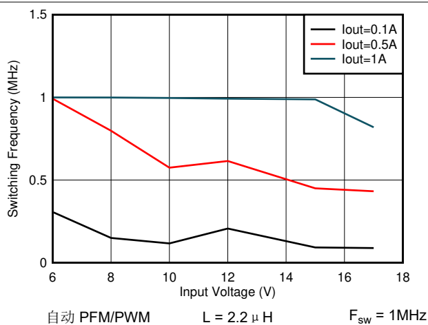
图 7-23. 开关频率与输入电压间的关系 V OUT = 5V
