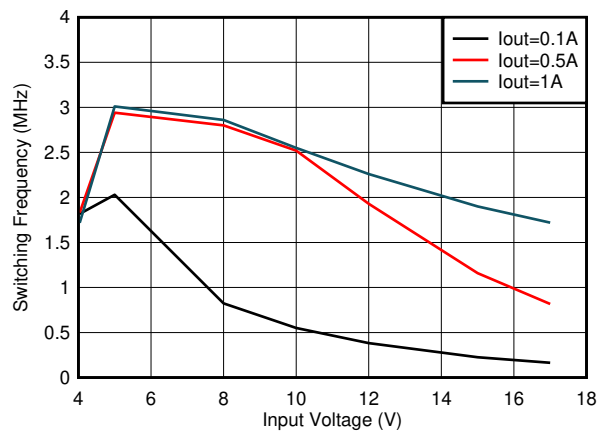
图 7-27. 开关频率与输入电压间的关系 V_{OUT} = 3.3V
