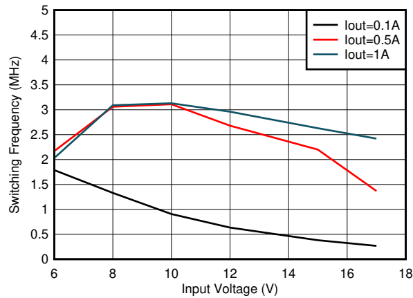
图 7-25. 开关频率与输入电压间的关系 V_{OUT} = 5V
