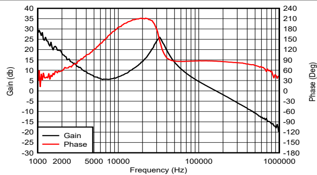
图 9-80. Bode Plot
