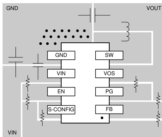
图 11-1. TPS629203 Layout
