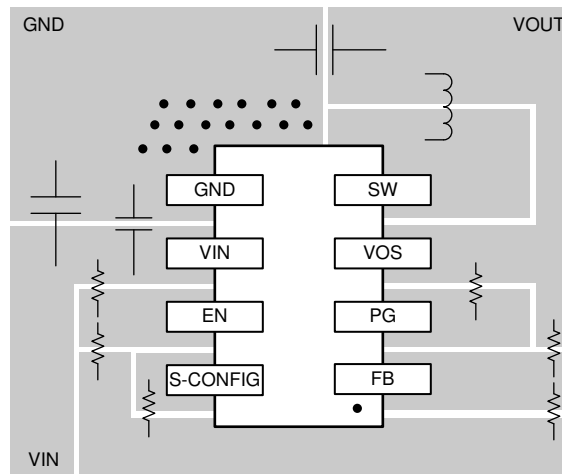
图 11-1. TPS629210 Layout
