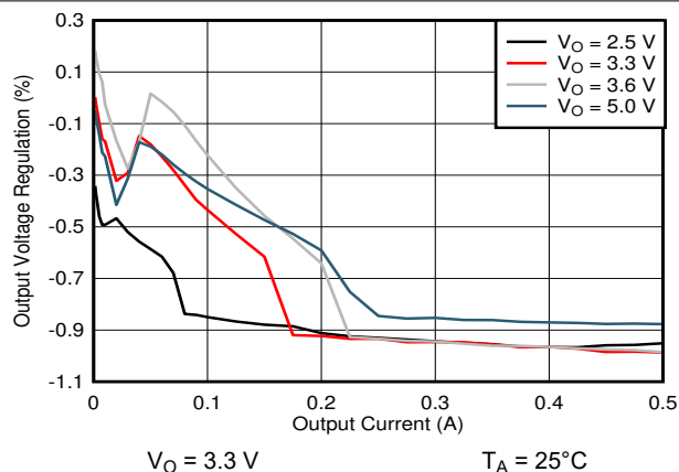
图 8-18. Load Regulation
