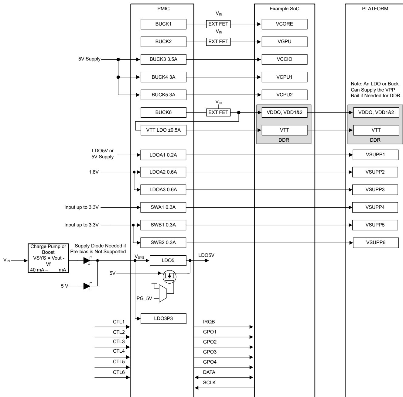
图 8-7. VIN 5-V Application
