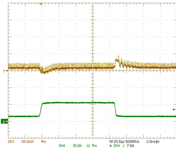
图 8-4. BUCK2 Controller Load Transient
