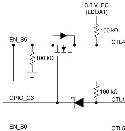
图 7-1. CTL Pin Implementation Option
