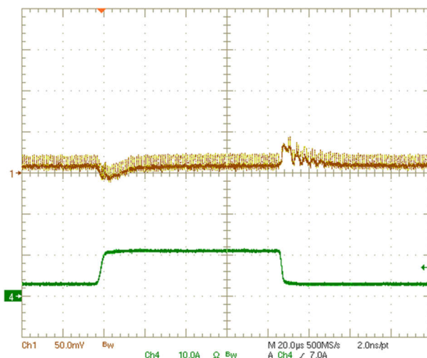
图 7-6. BUCK2 Load Transient
