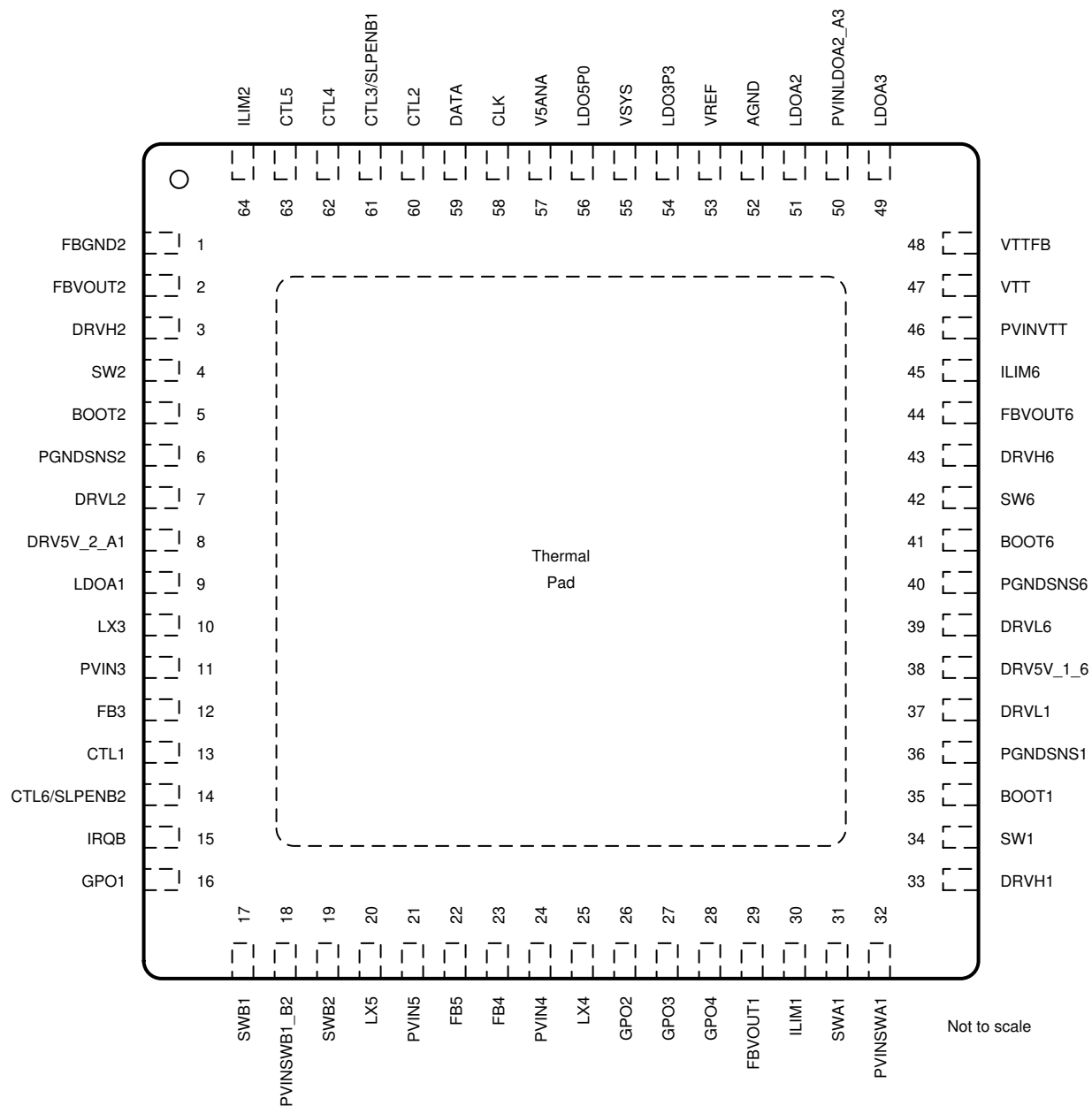
图 4-1. 64-pin RSK VQFN (Top View)
