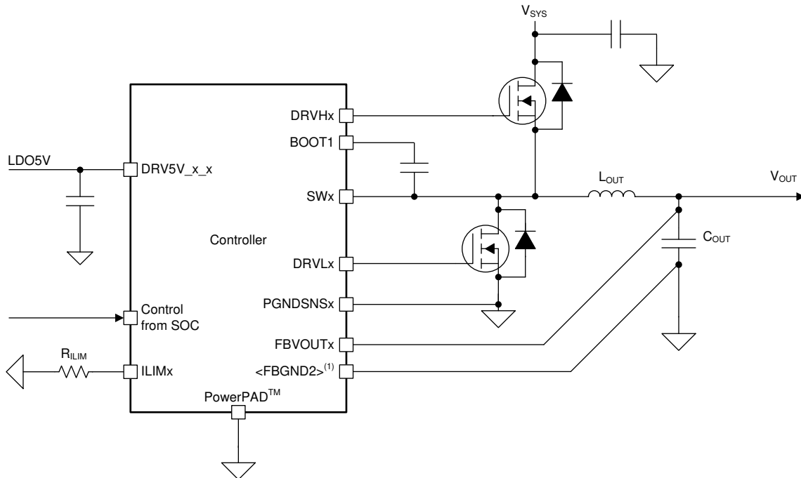
图 7-3. Controller Diagram
