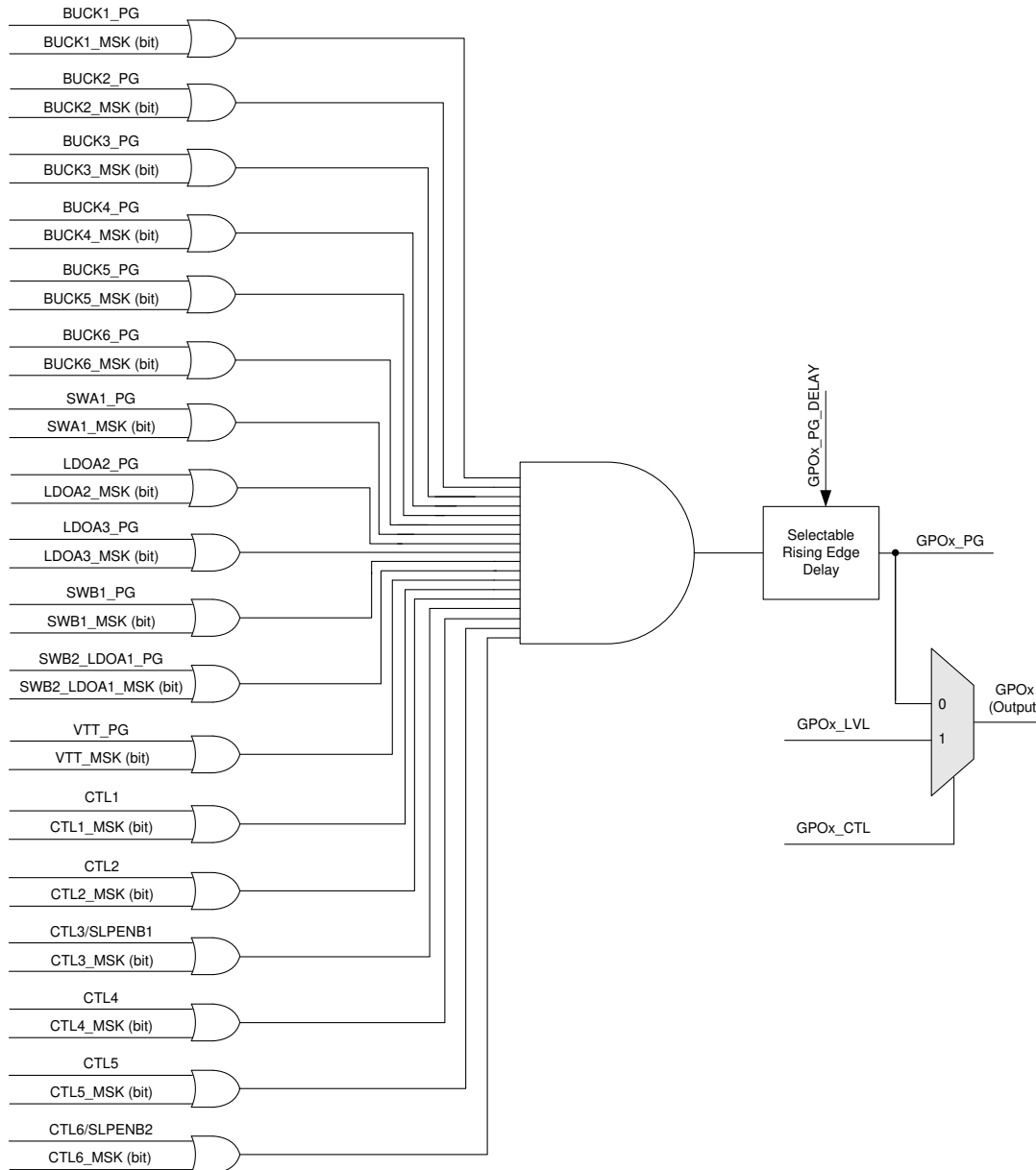
图 6-6. Power Good Tree
