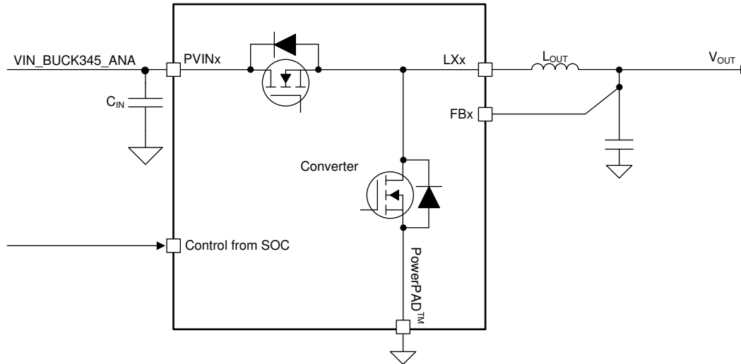
图 7-5. Converter Diagram
