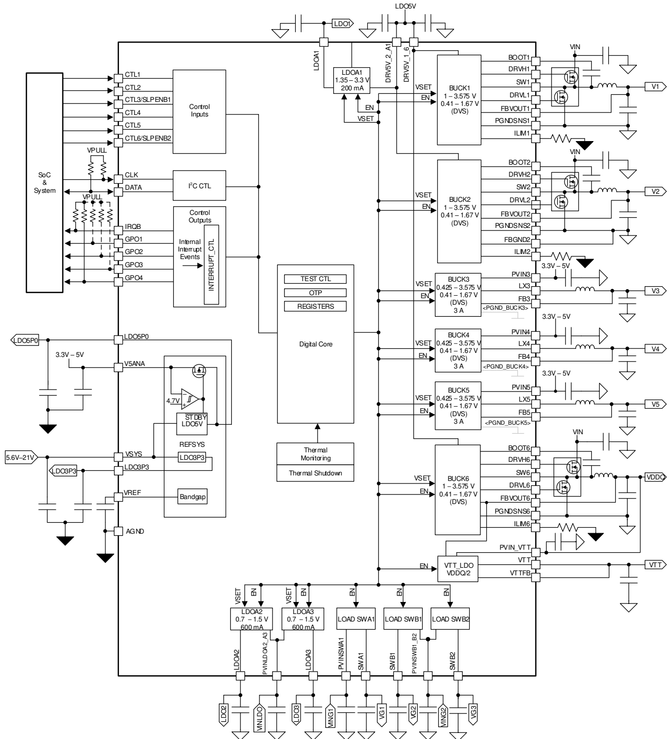
PMIC 功能方框图
