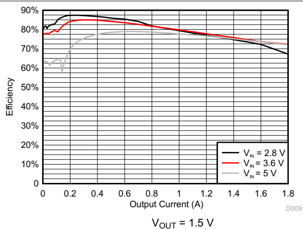
图 8-6. DCDC3 Efficiency
