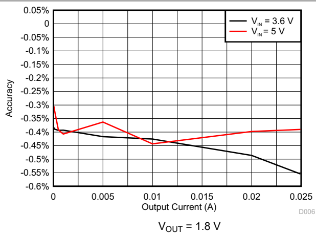
图 6-6. DCDC6 Accuracy
