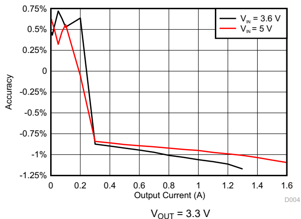
图 6-4. DCDC4 Accuracy
