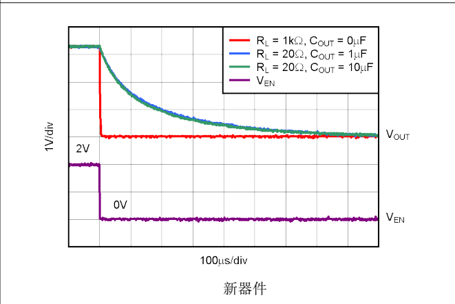
图 5-42. TPS73133 关断响应
