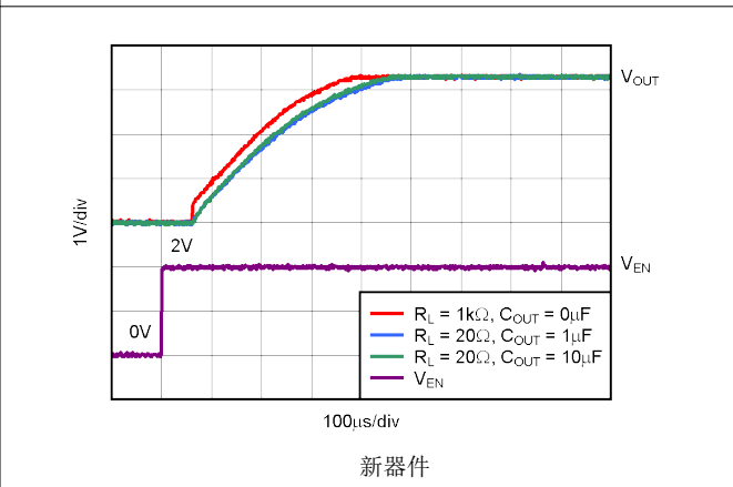
图 5-40. TPS73133 导通响应
