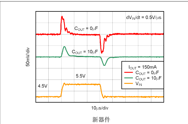
图 5-38. TPS73133 线路瞬态响应
