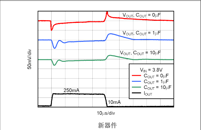
图 5-36. TPS73233 负载瞬态响应
