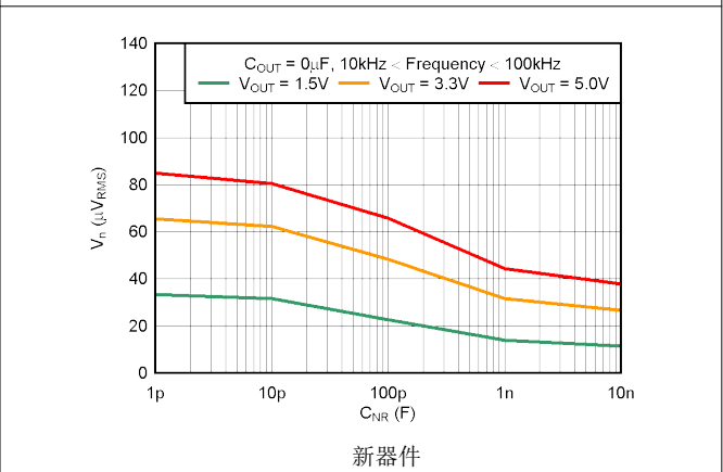
图 5-34. RMS 噪声电压与 C_{NR} 间的关系
