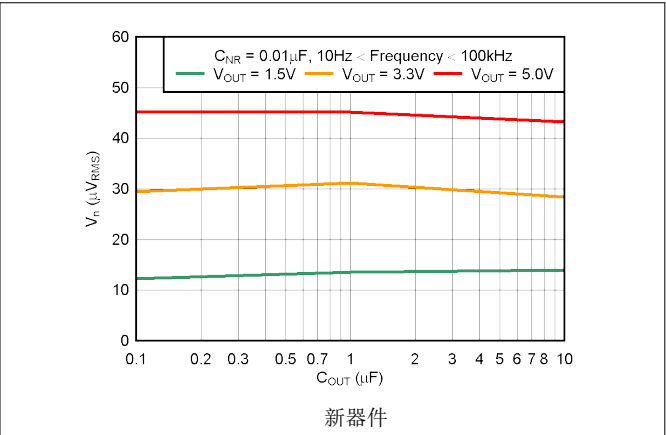
图 5-32. RMS 噪声电压与 C_{OUT} 间的关系
