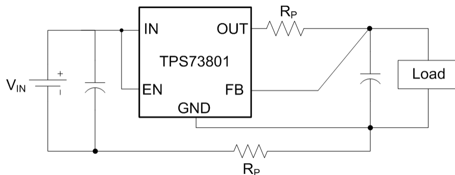
图 6-2. Kelvin Sense Connection
