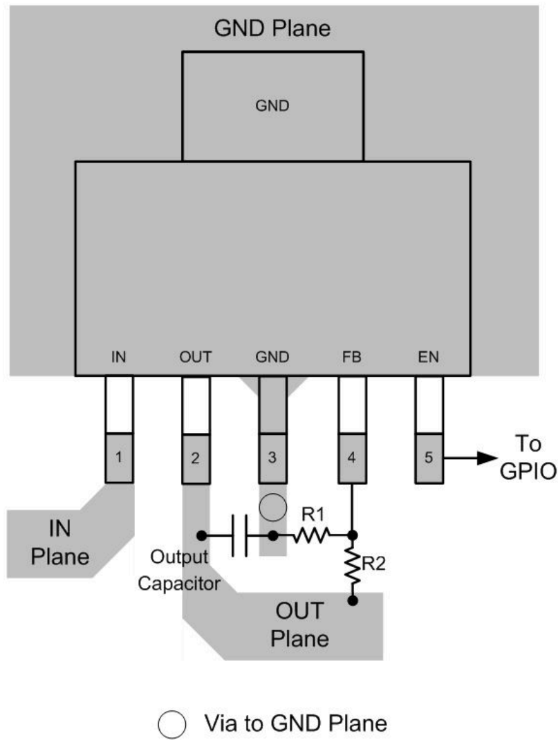
图 7-3. SOT-223 Layout Example (DCQ)
