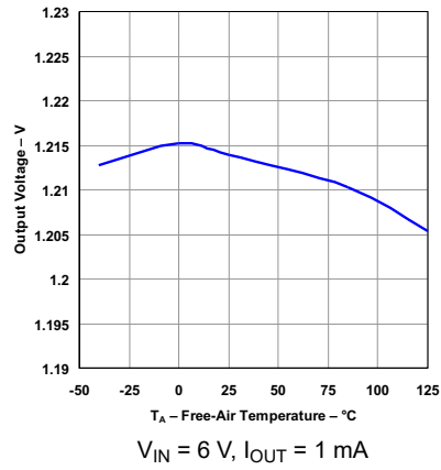
图 5-4. Output Voltage vs Temperature
