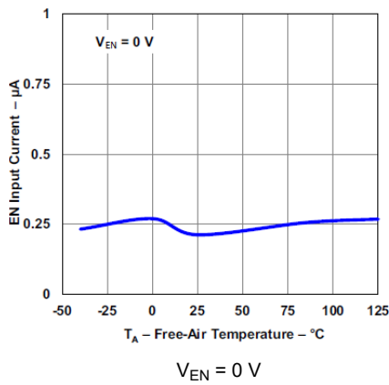
图 5-9. EN Input Current vs Temperature
