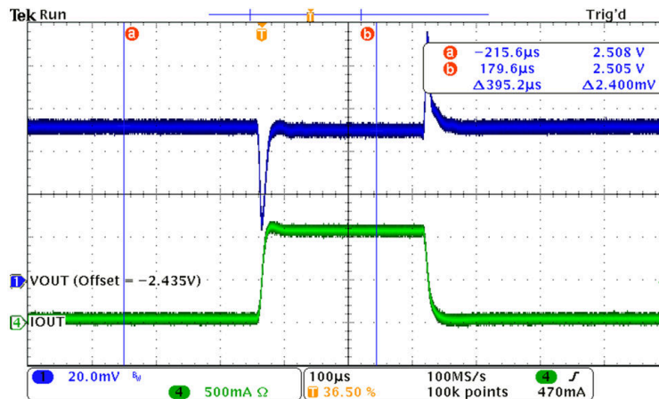
图 7-2. 1-A Load Transient Response
