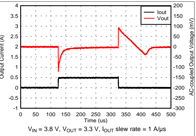
图 26. 3.3-V, 1-mA to 500-mA Load Transient
