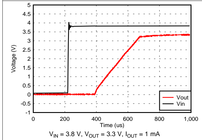
图 29. VIN Power-Up
