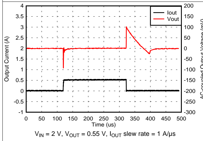
图 27. 0.55-V, 1-mA to 500-mA Load Transient
