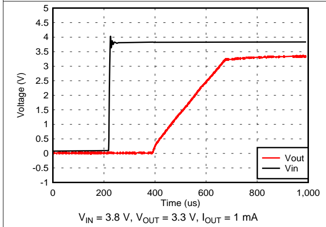
图 29. VIN Power-Up
