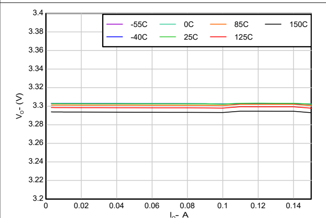
图 5-4. TPS76333 输出电压与输出电流间的关系 (新芯片)
