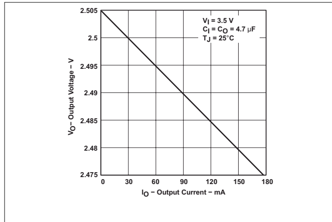
图 5-1. TPS76325 输出电压与输出电流间的关系 (旧芯片)
