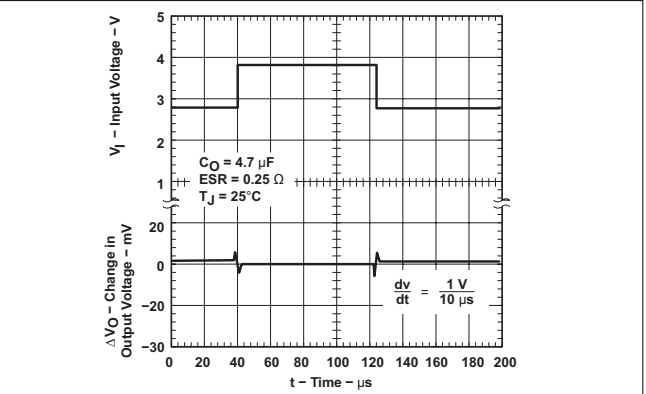
图 5-24. TPS76318 线路瞬态响应 (旧芯片)
