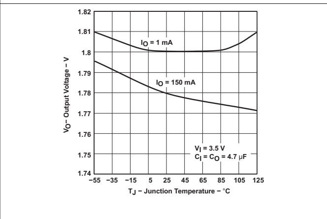
图 5-6. TPS76318 输出电压与自然通风温度间的关系 (旧芯片)
