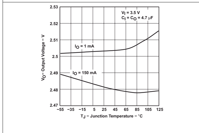
图 5-5. TPS76325 输出电压与自然通风温度间的关系 (旧芯片)
