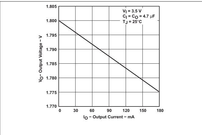
图 5-2. TPS76318 输出电压与输出电流间的关系 (旧芯片)
