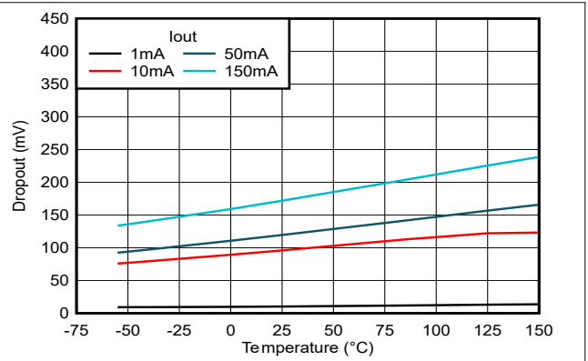
图 5-20. TPS76333 压降电压与温度之间的关系 (新芯片)
