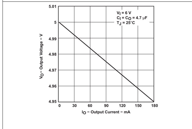
图 5-3. TPS76350 输出电压与输出电流间的关系 (旧芯片)
