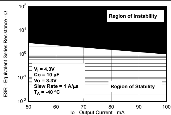
图 5-64. 典型稳定性 ESR 区域与输出电流间的关系（新芯片）
