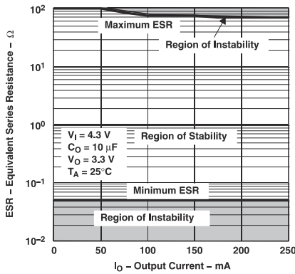
图 5-54. 典型稳定性 ESR 区域与输出电流间的关系（新芯片）
