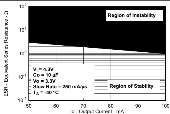
图 5-65. 典型稳定性 ESR 区域与输出电流间的关系（新芯片）
