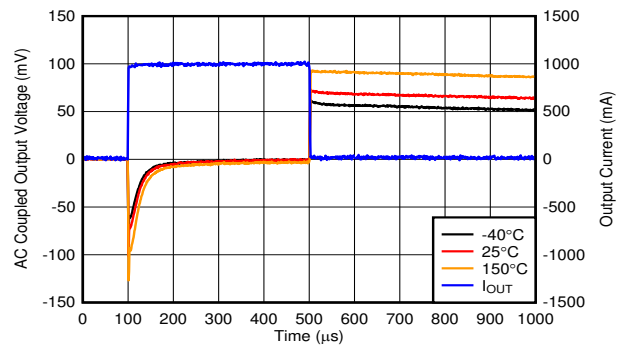
图 6-20. Load Transient vs Temperature
