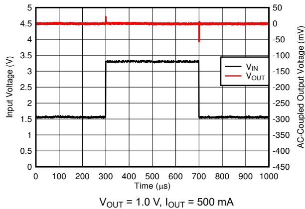
图 6-19. V_{IN} Transient
