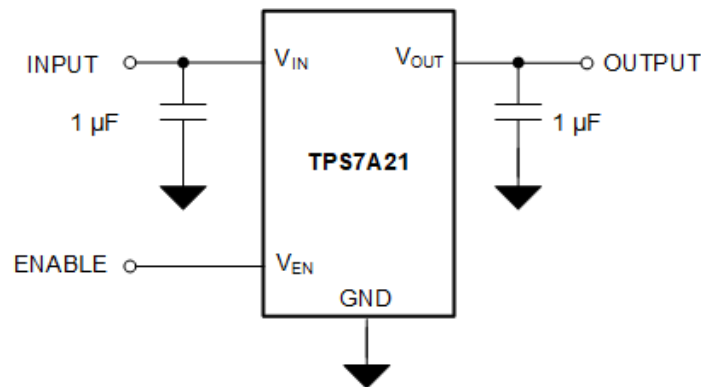
简化原理图
