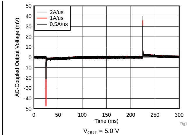
图 48. Load Transient vs Slew Rate
