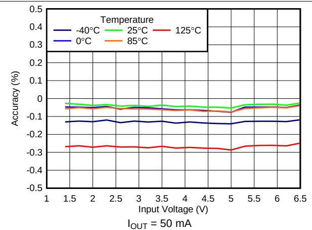
图 17. Line Regulation
