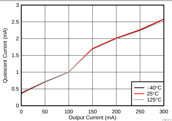
图 2. Quiescent Current vs Output Current (TPS7B7701-Q1)
