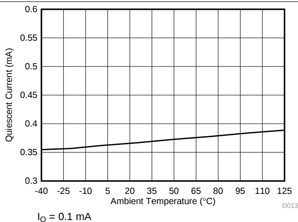
图 5. Quiescent Current vs Ambient Temperature (TPS7B7701-Q1)
