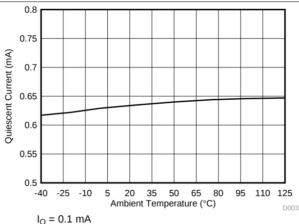
图 4. Quiescent Current vs Ambient Temperature (TPS7B7702-Q1)
