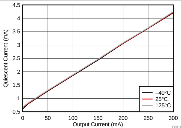
图 1. Quiescent Current vs Output Current (TPS7B7702-Q1)
