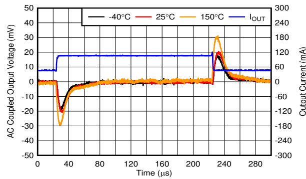
图 8-7. Transient Response
