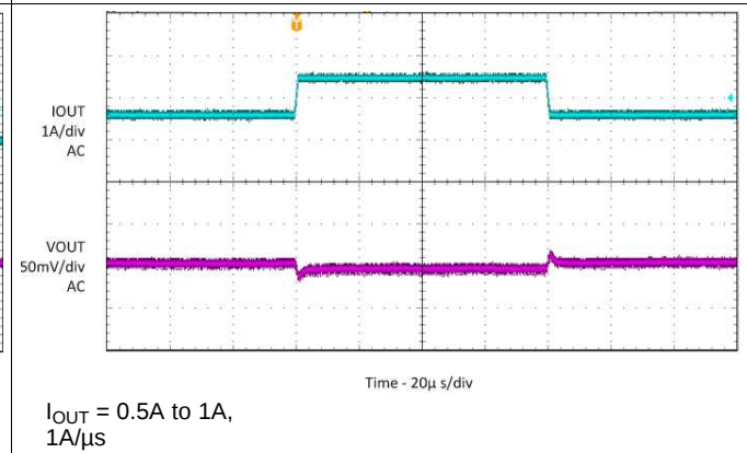
图 27. Load Transient
