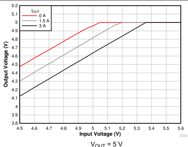
图 7-9. Voltage Dropout
