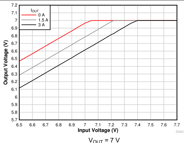
图 7-11. Voltage Dropout
