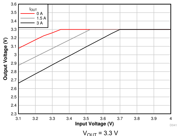
图 7-7. Voltage Dropout
