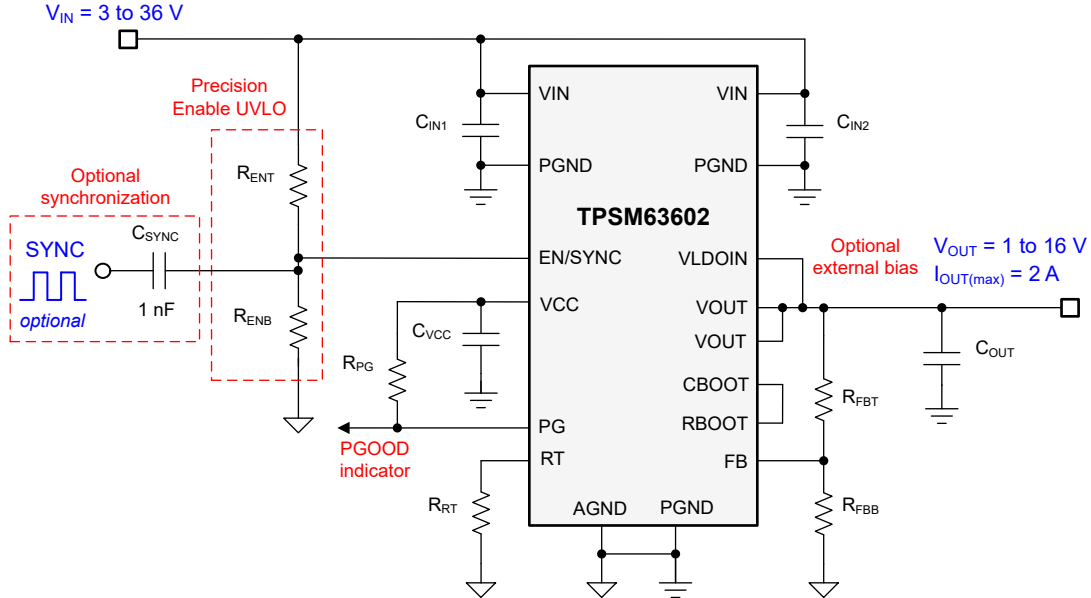
图 8-1. 输入工作电压范围为 3V 至 36V 的 TPSM63602 原理图
