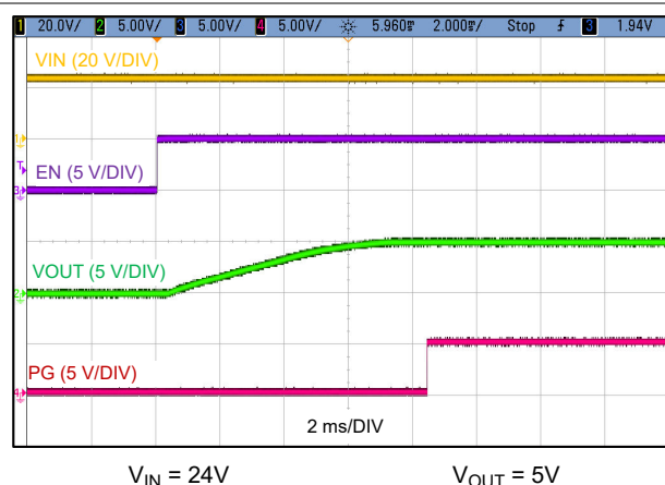
图 9-2. 启动波形
