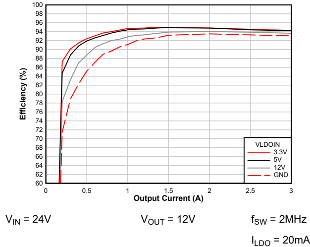
图 8-9. 通过 VLDOIN 实现的效率提升 ( V_{OUT} = 12V )
