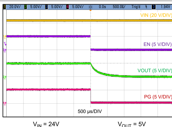
图 9-3. 关断波形
