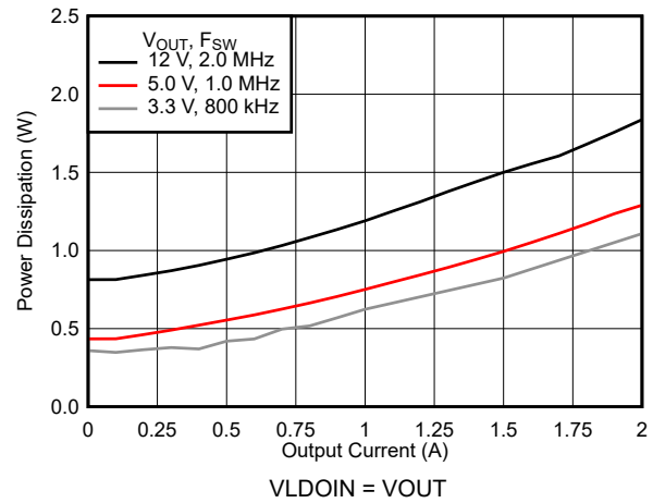
图 7-18. 功率耗散
