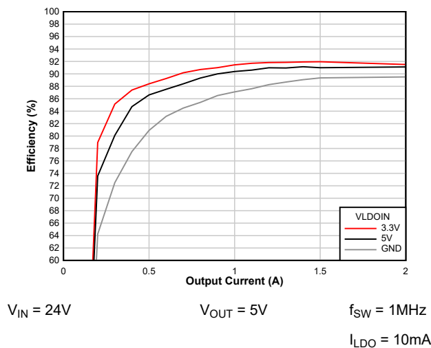
图 8-8. 通过 VLDOIN 实现的效率提升 ( V_{OUT} = 5V )
