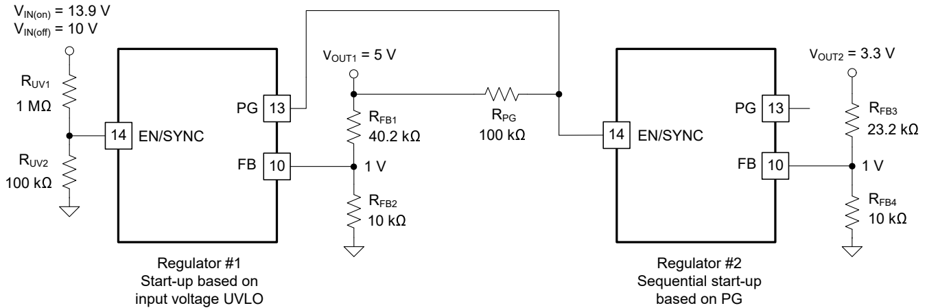
图 8-6. 使用 PG 和 EN/SYNC 的 TPSM63602 时序控制实现
