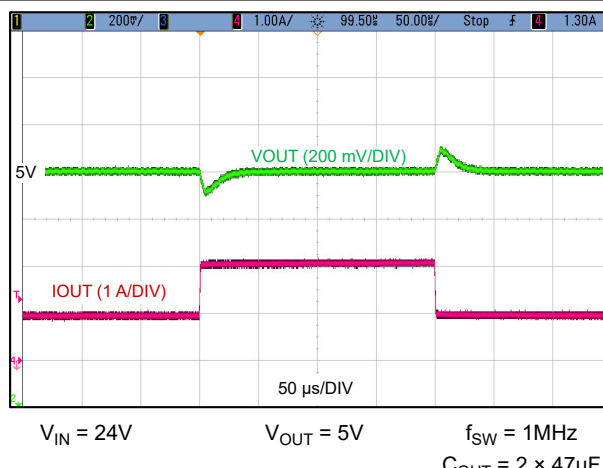
图 9-5. 负载瞬态 (1A 至 2A, 1A/μs)
