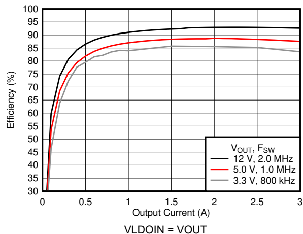
图 7-19. 效率
