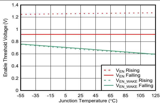
图 7-5. 使能阈值
