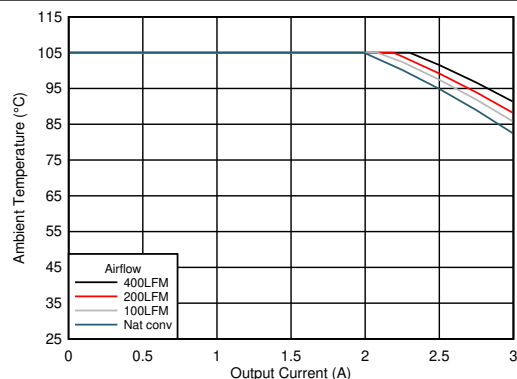
图 7-12. 安全工作区
