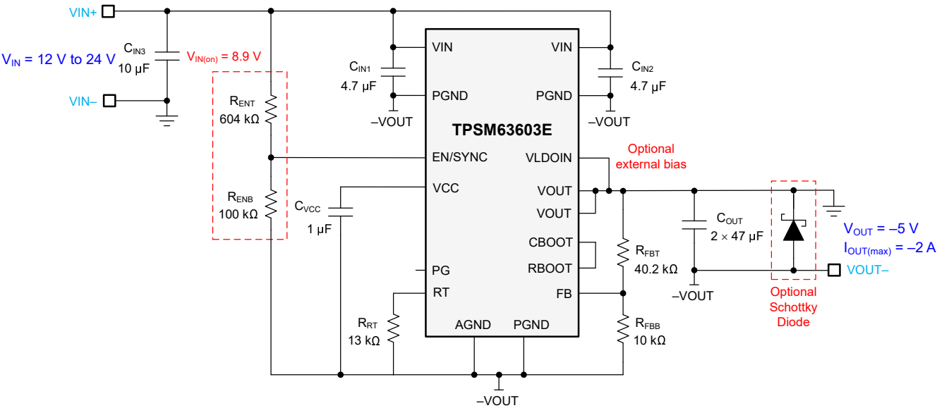
图 9-12. 电路原理图
