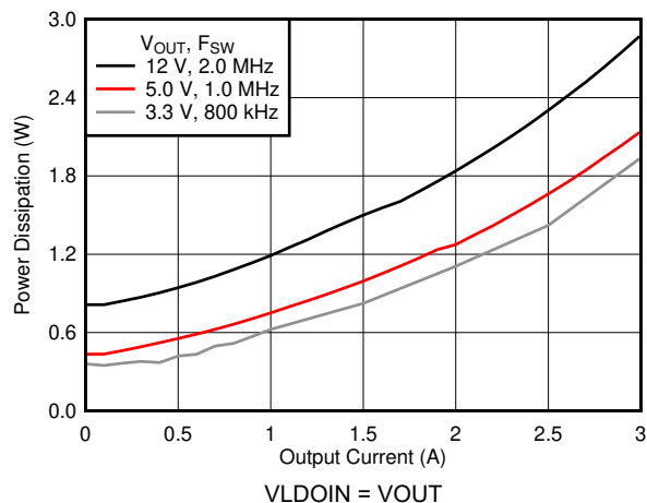
图 7-20. 功率耗散
