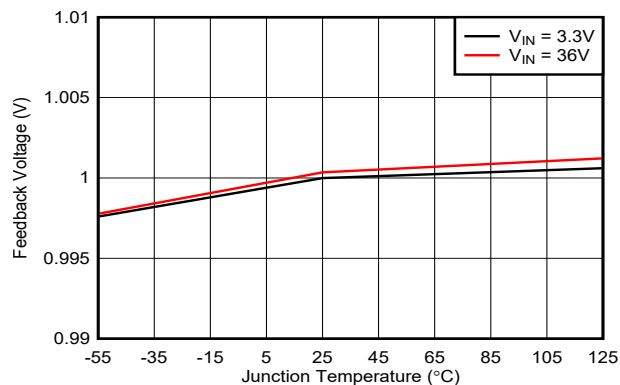
图 7-2. 反馈电压
