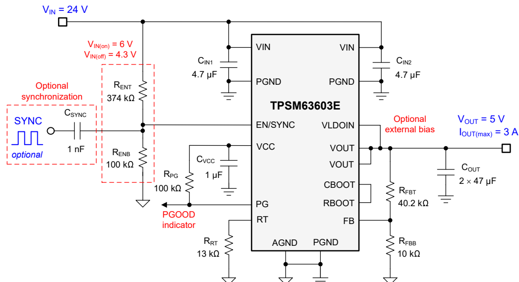
图 9-1. 电路原理图
