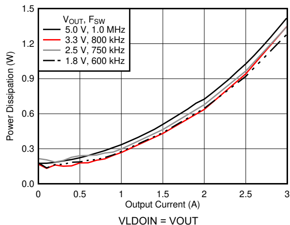
图 7-8. 功率耗散
