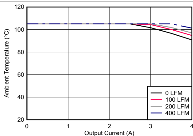
图 7-18. 安全工作区 ( V_{OUT} = 5V , F_{SW} = 1MHz )
