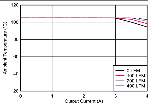
图 7-17. 安全工作区 ( V_{OUT} = 3.3V , F_{SW} = 750kHz )
