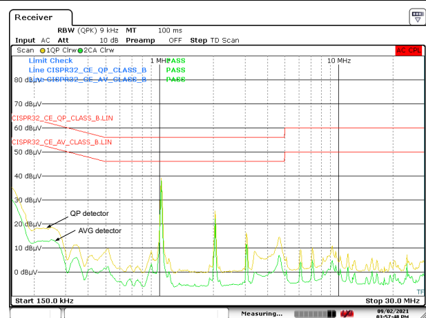
图 9-7. CISPR 32 B 类传导发射: V_{IN} = 24V
