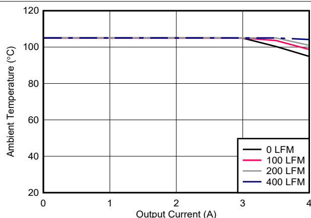
图 7-16. 安全工作区 ( V_{OUT} = 2.5V , F_{SW} = 500kHz )
