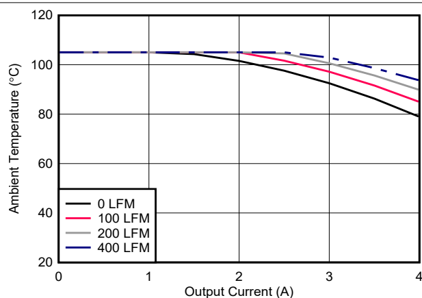
图 7-19. 安全工作区 ( V_{OUT} = 12V , F_{SW} = 2MHz )
