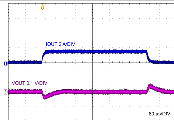
图 9-14. 负载瞬态, 0A 至 1.5A
