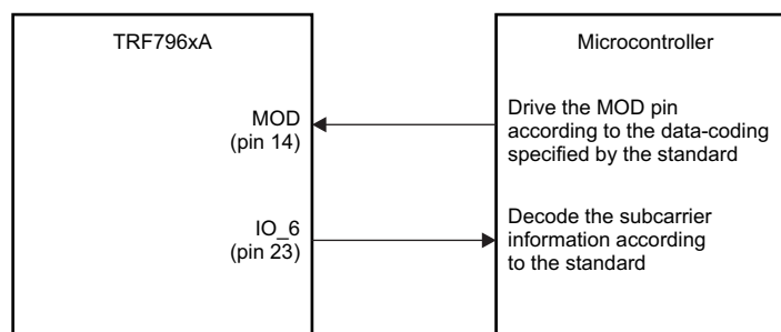
图 6-28. Control of RF Modulation Using MOD
