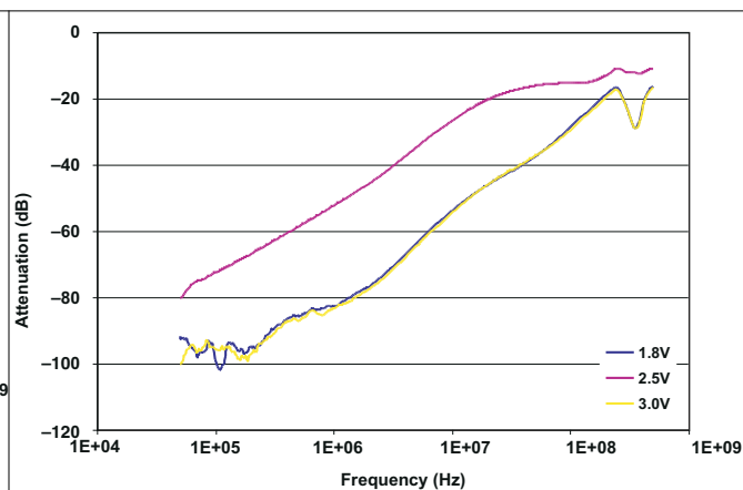
图 6-8. Crosstalk
