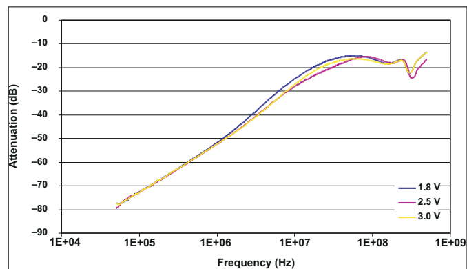
图 6-7. OFF Isolation
