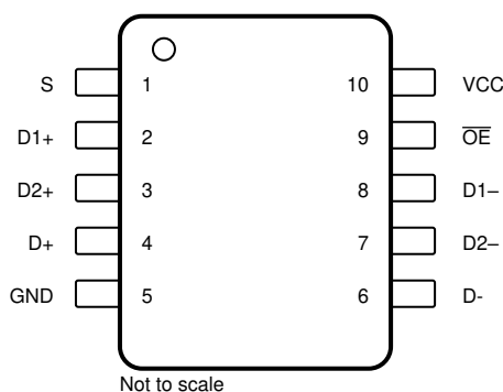
图 4-2. DGS Package 10-Pin VSSOP Top View
