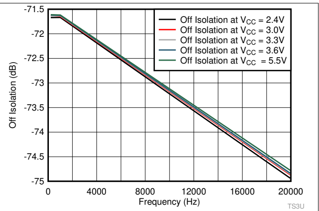
图 4. Off Isolation
