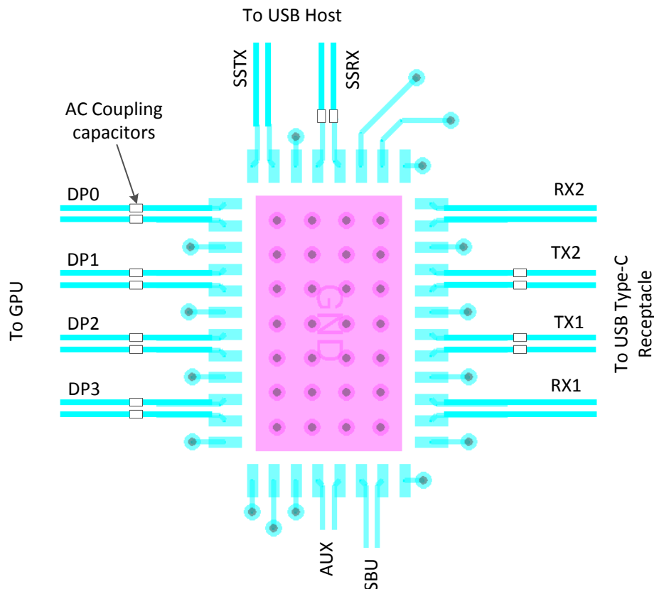
图 10-1. Layout Example
