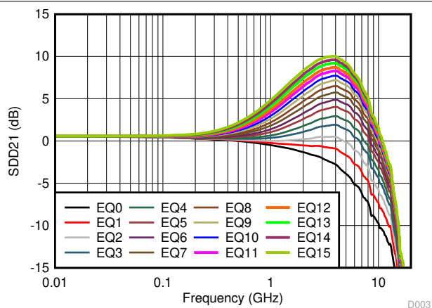
图 6-3. USB TX EQ Settings Curves
