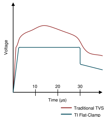
对 8 \mu s 至 20 \mu s 浪涌事件的电压钳位响应
