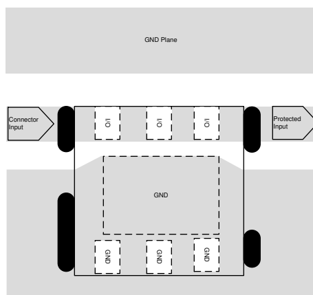
图 9-3. TVS2200 Layout
