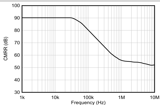
图 5-14. CMRR 与频率间的关系 (新裸片)
