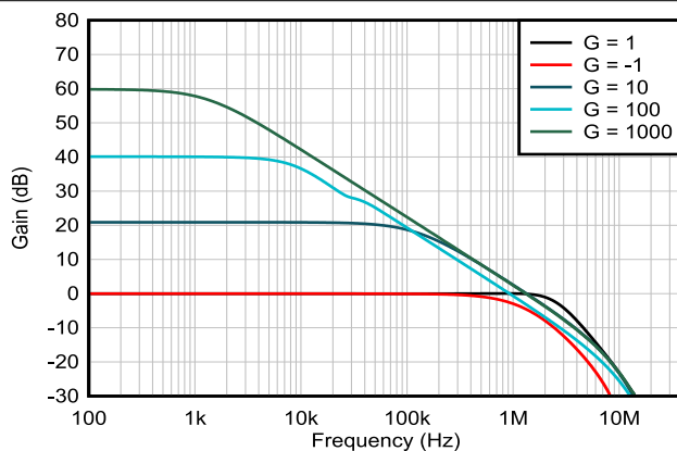
图 5-12. 闭环增益与频率间的关系 (新裸片)
