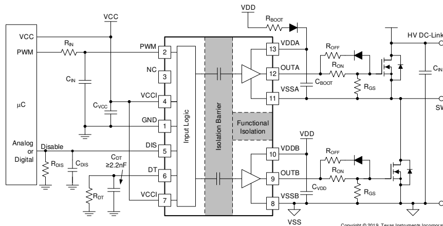
功能方框图
