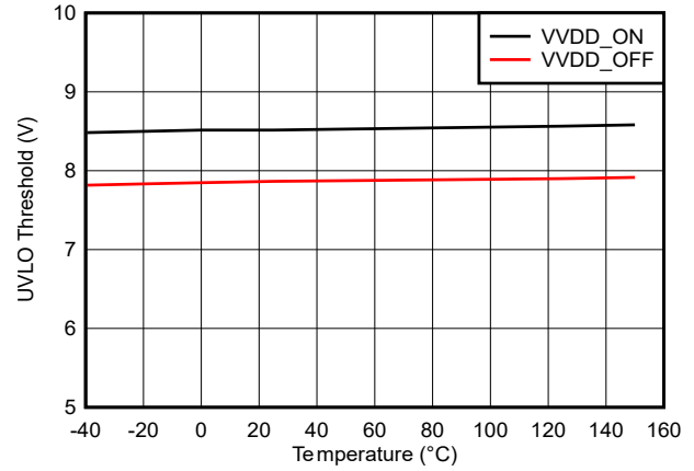
图 5-17. VDD 8V UVLO 阈值与温度之间的关系
