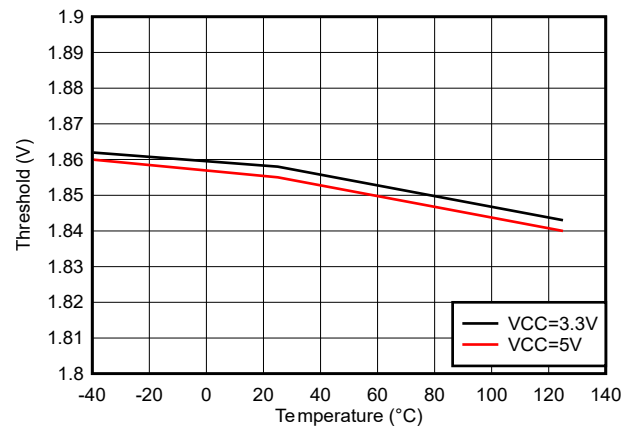
图 5-21. IN/DIS 高阈值
