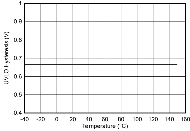
图 5-18. VDD 8V UVLO 迟滞与温度之间的关系
