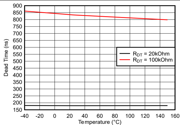
图 5-22. 死区时间与温度之间的关系 ( R_{DT} = 20k\Omega 和 100k\Omega )
