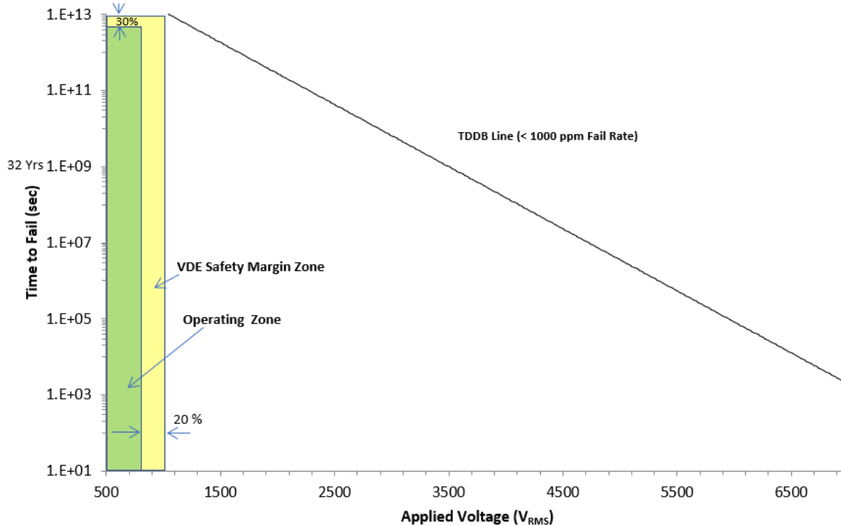
图 5-3. 基本隔离电容器寿命预测
