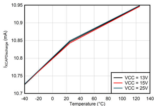
图 6-16. I_{XCAPDischarge} vs Temperature
