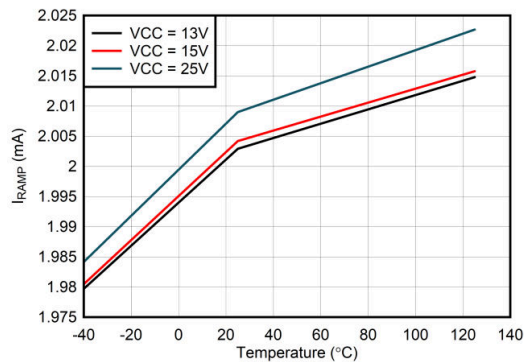
图 6-6. I_{RAMP} vs Temperature
