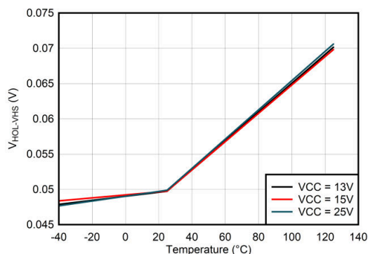
图 6-22. V_{HOL-V_{HS}} vs Temperature
