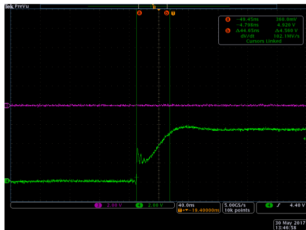
图 8-3. HO Rise Time
