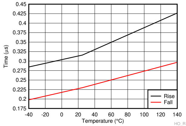
图 6-27. HO Rise &amp; Fall Time
