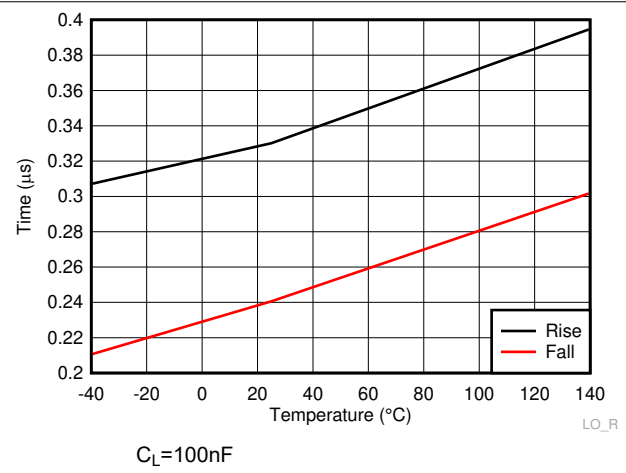
图 6-26. LO Rise & Fall Time
