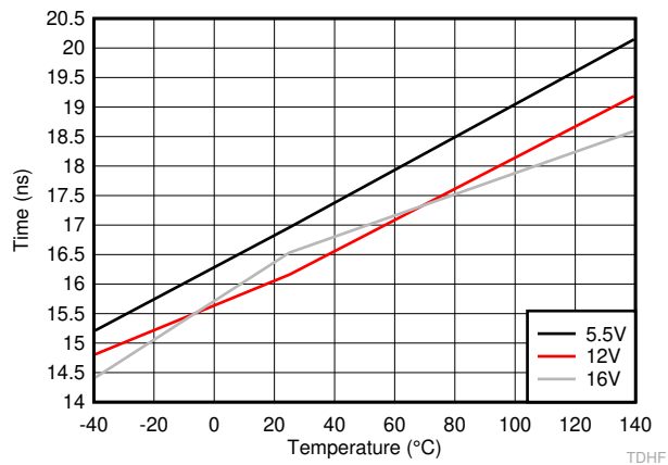
图 6-27. HO Rise &amp; Fall Time
