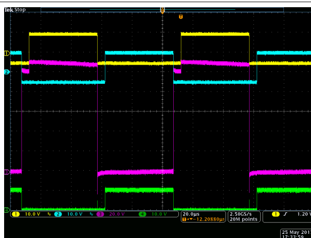
A. V_{DD} = 10\text{ V} V_{in} = 100\text{ V} C_L = 1\text{ nF} Ch1 = HI Ch2 = LI Ch3 = HO Ch4 = LO
