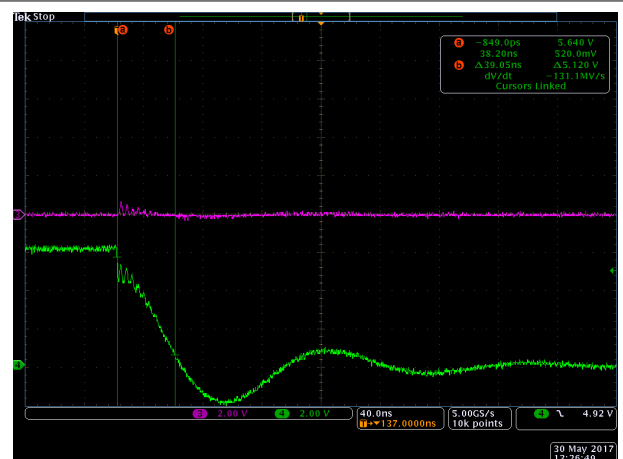
图 8-4. HO Fall Time
