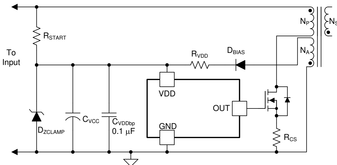
图 8-1. VDD Protection
