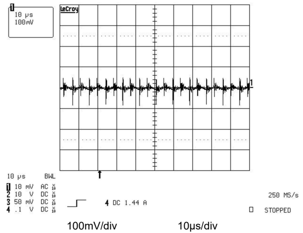
图 8-9. 满载条件下的输出电压纹波
