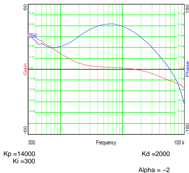
图 7-12. Bode Plot
