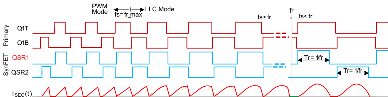
图 6-10. LLC Waveforms
