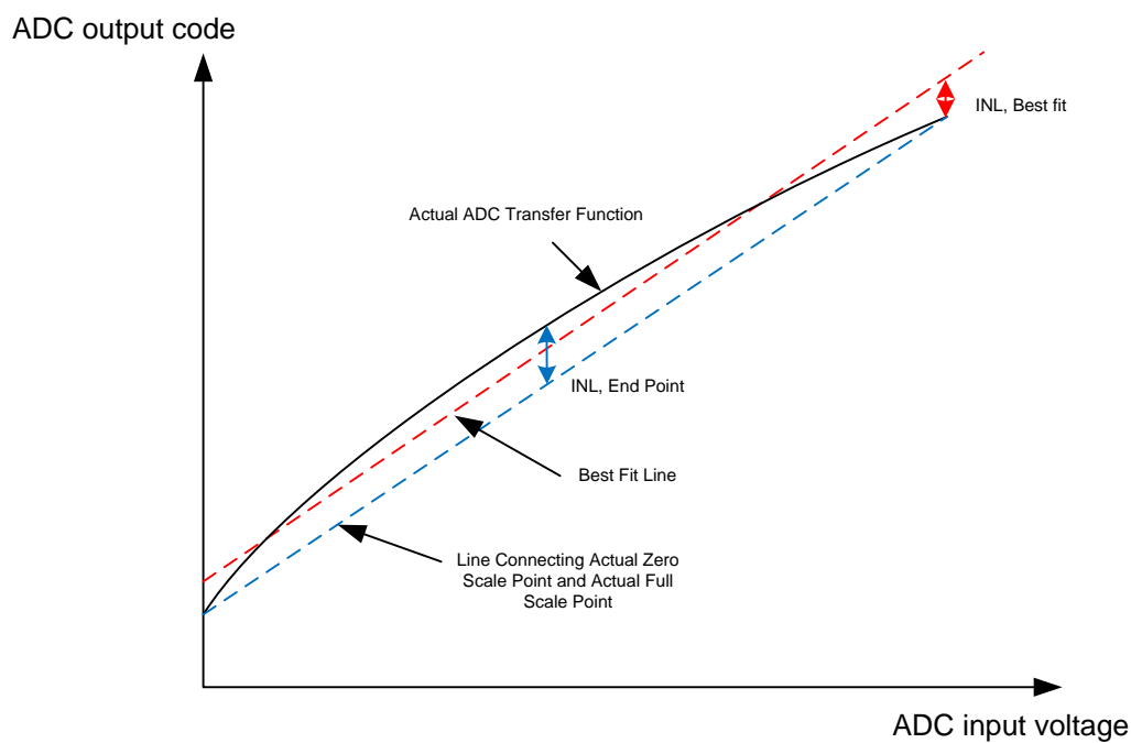
图 5-3. Best Fit INL and End Point INL
