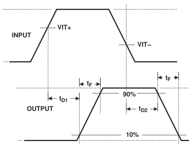
图 8-1. Timing Diagram
