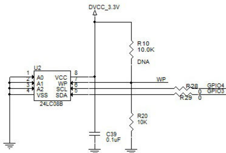
图 9-5. External EEPROM
