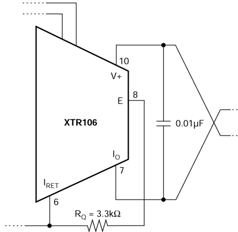
(1) 如需在没有外部晶体管的情况下运行，在引脚 6 和引脚 8 之间连接一个 3.3kΩ 电阻器。有关对性能的讨论，请查看文本。
